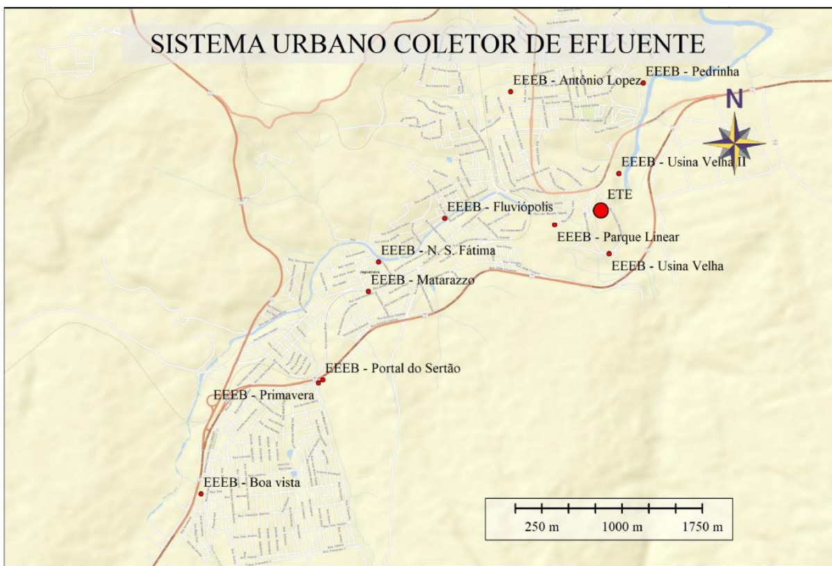
Figura 09 - Localização das ETEB e da ETE.
